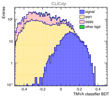
Fig. 6 Pattern Fill
