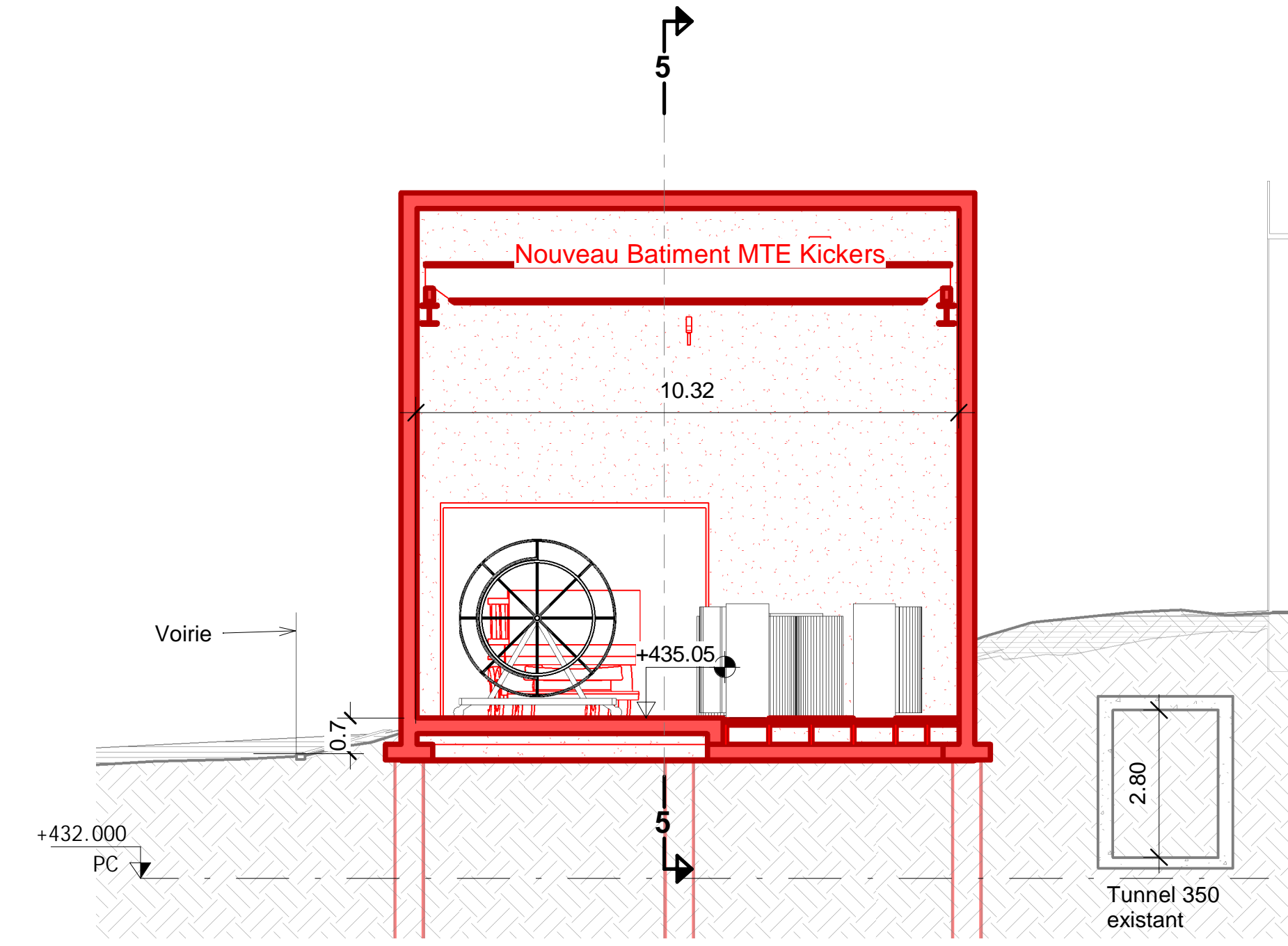
Section 1 Sc. 1 : 100
