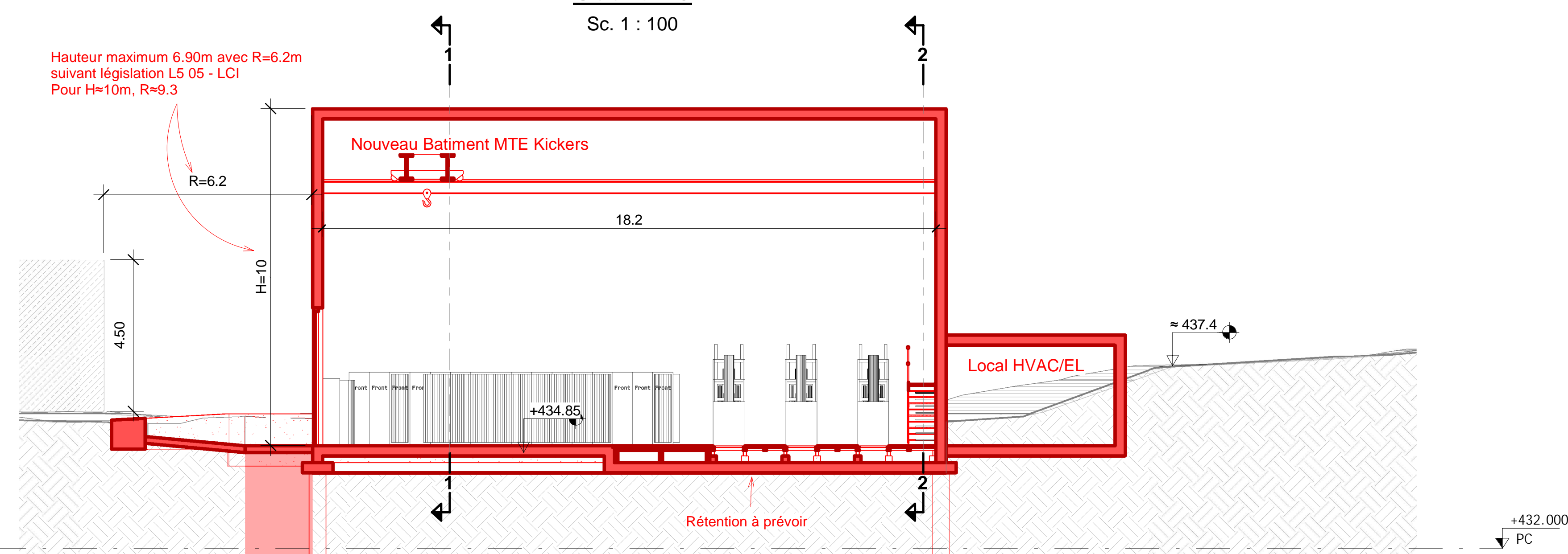
Section 5 Sc. 1 : 100
