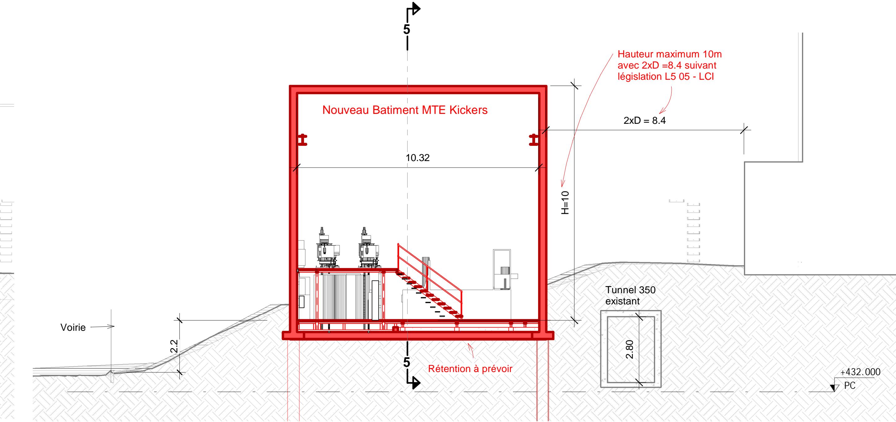
Section 2 Sc. 1 : 100
