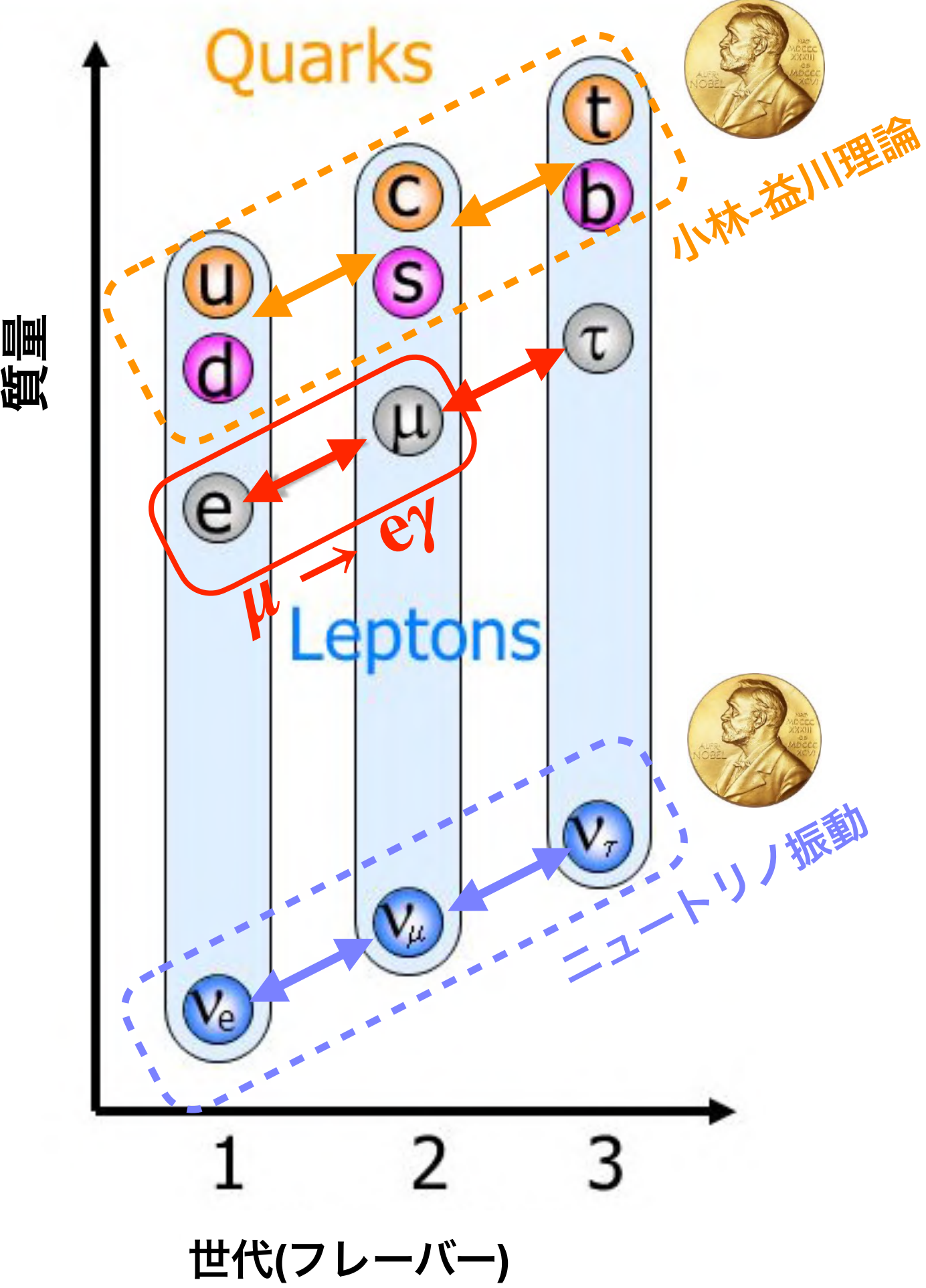
物質粒子(クォークとレプトン)の3世代構造
