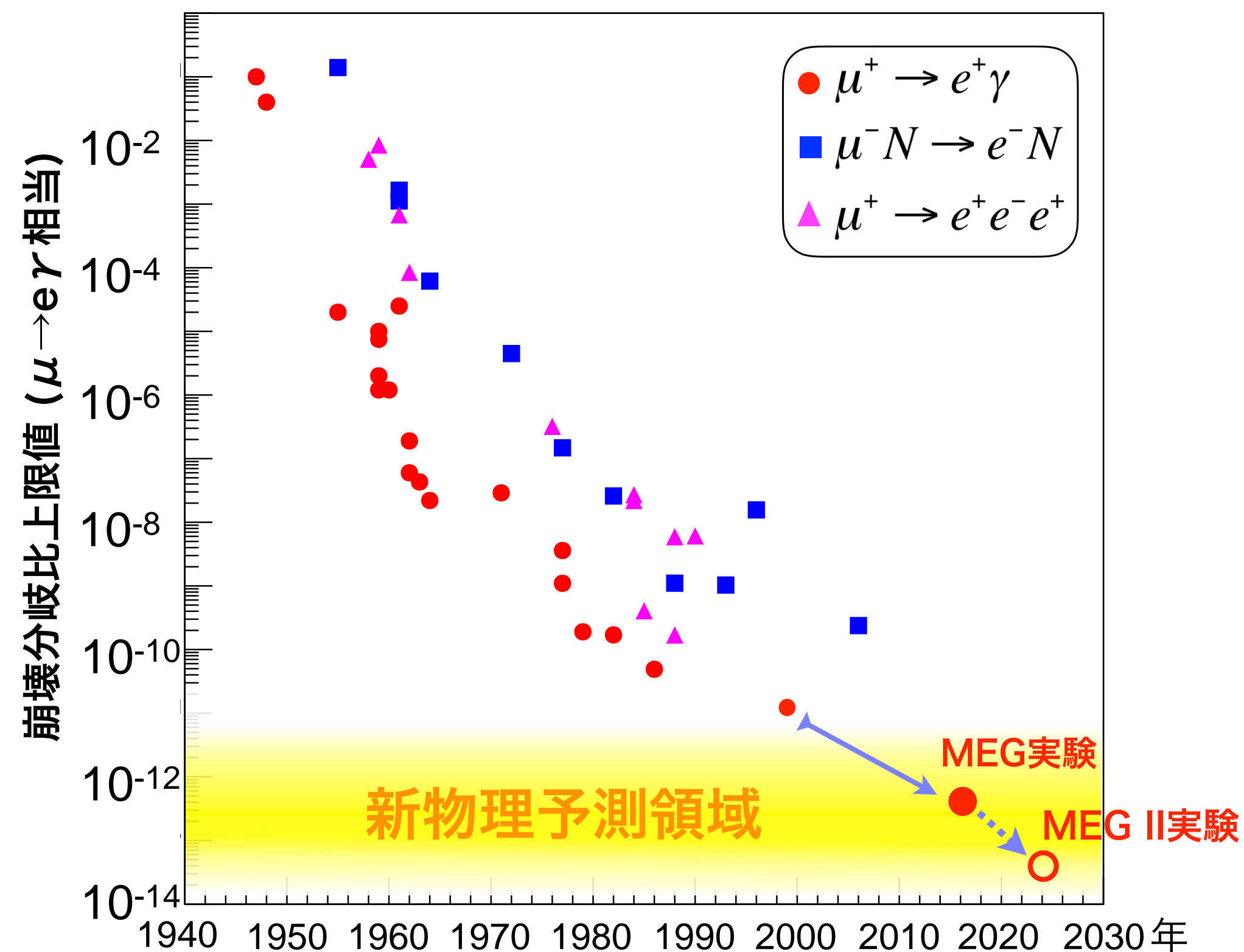
\mu \rightarrow e\gamma 探索実験の歴史
