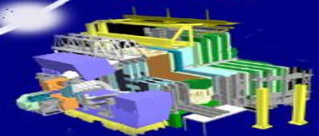
LHCb
