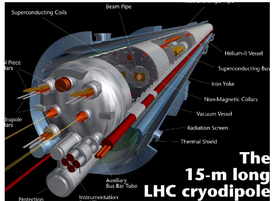
Υπεραγώγιμο δίπολο του LHC
