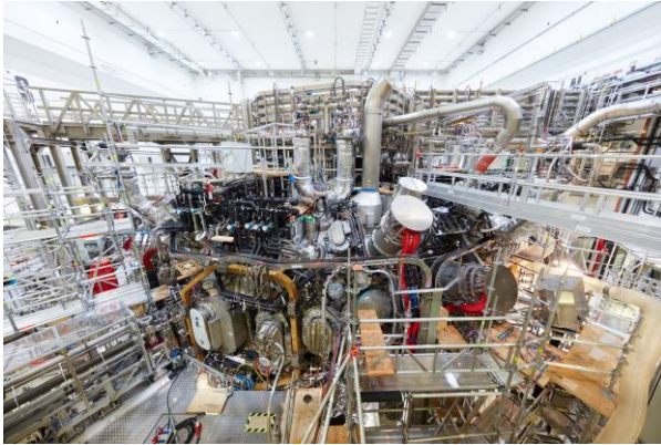
Fig. 1: Stellarator Wendelstein W7-X
