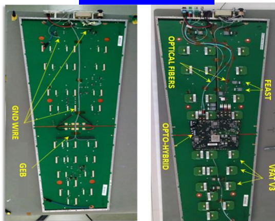
GE1/1 GEB & OH
