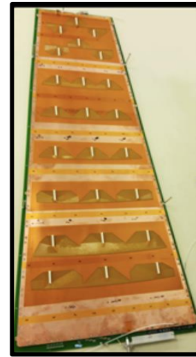
GE1/1-V
