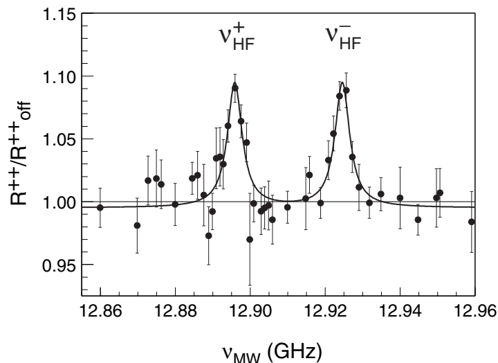
Mikrohullámú frekvencia-spektrum
