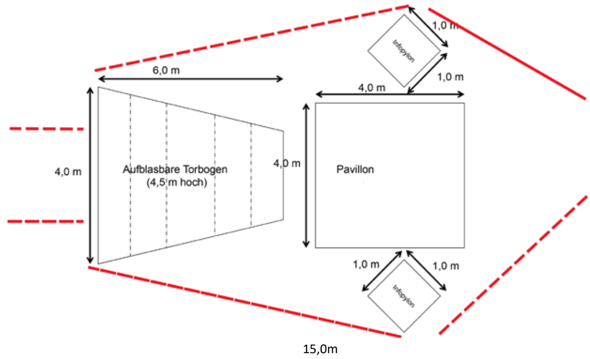
Aufbau Skizze
