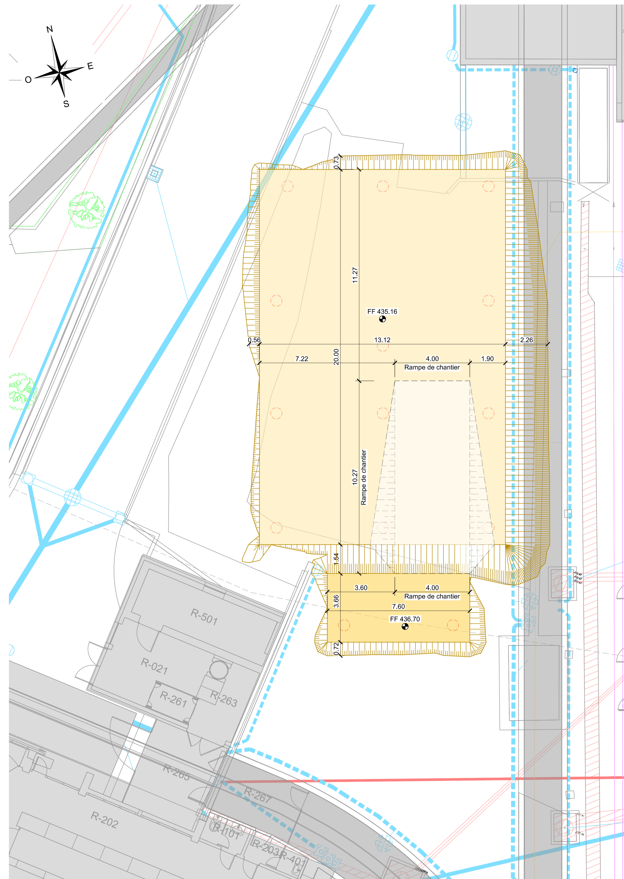
SITUATION PRE-TERRASSEMENT POUR FORAGE DES PIEUX 1/100
