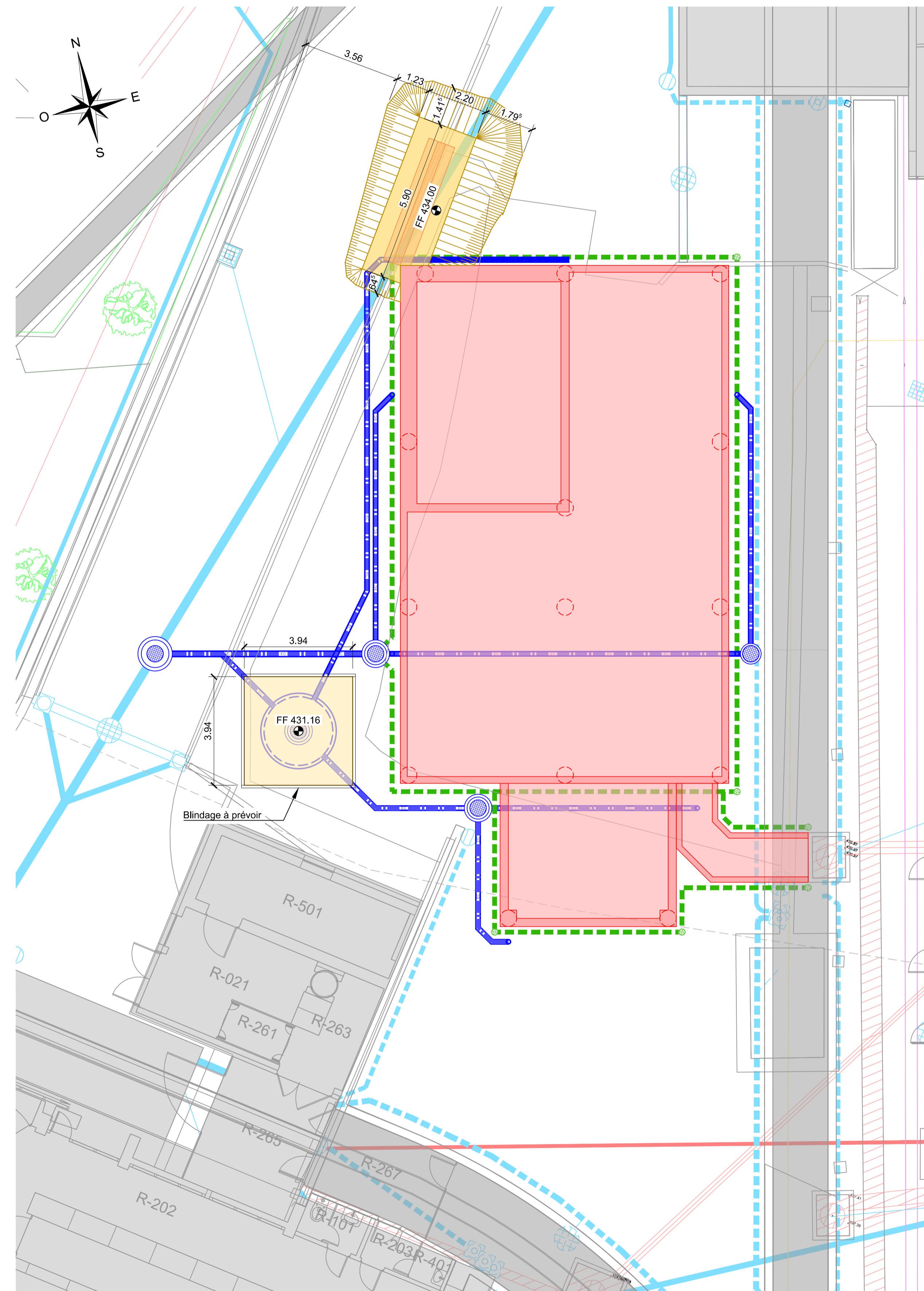
SITUATION TERRASSEMENT ETAPE 2 1/100
