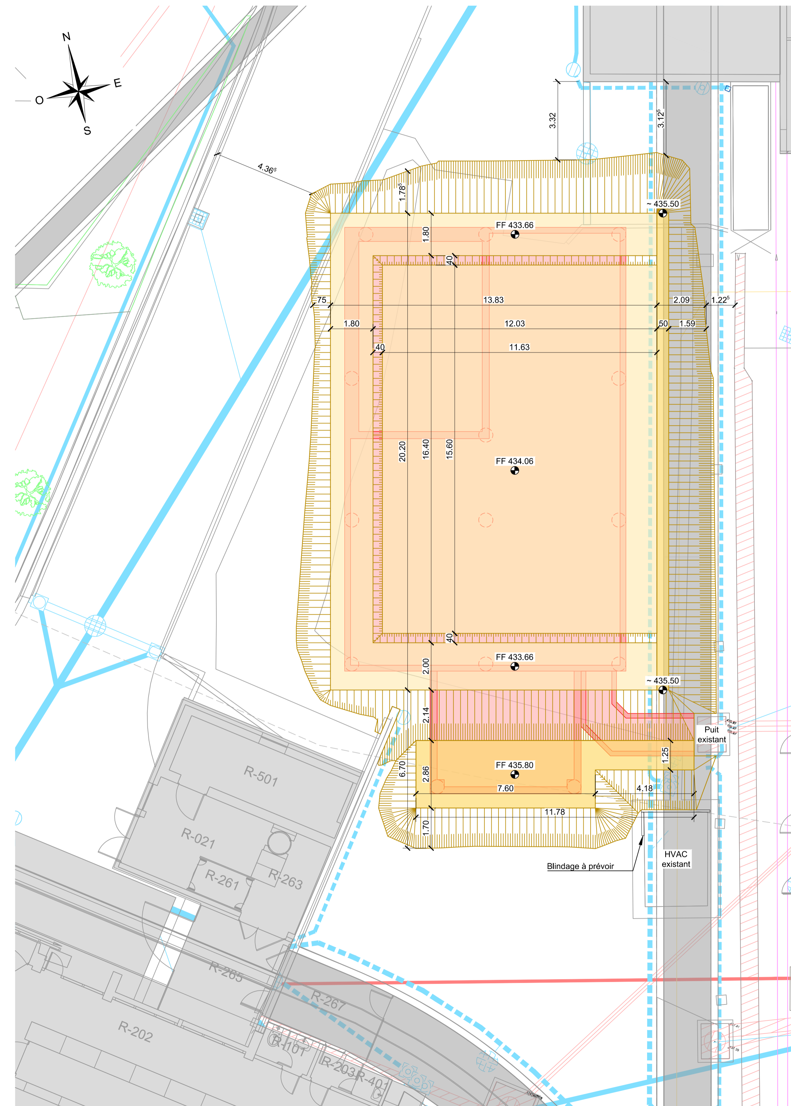
SITUATION TERRASSEMENT ETAPE 1 1/100
