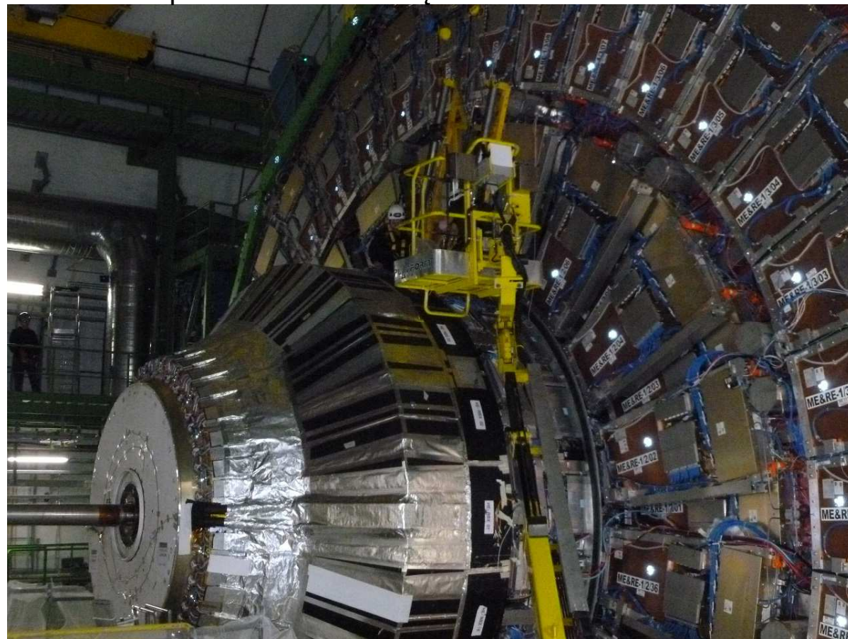
CERN “Kompaktiškas” miuonų solenoido detektorius
