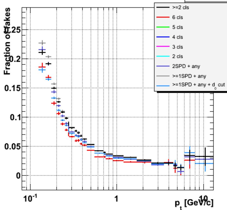
MC Hijing LHC11a4_bis
