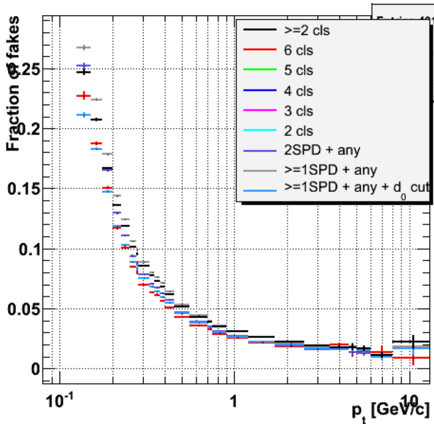
MC Hijing LHC11a4
