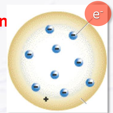
'Rosinenkuchen' Modell des Atoms (1904)
