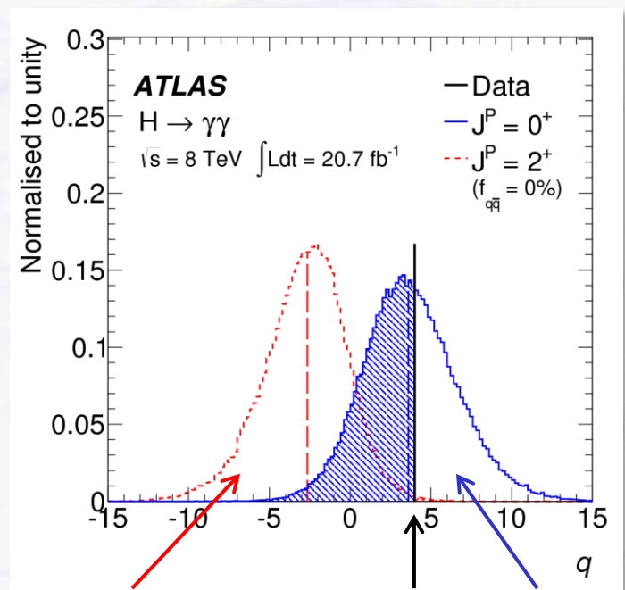
Erwartung für 2^+ Messung Erwartung für 0^+
