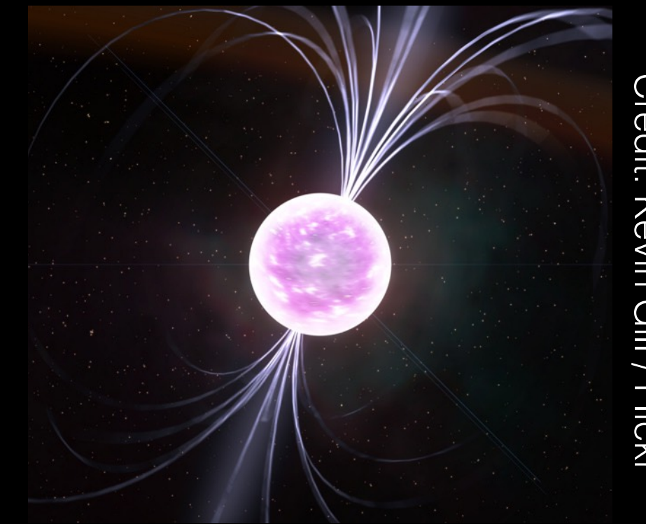
Pulsars
