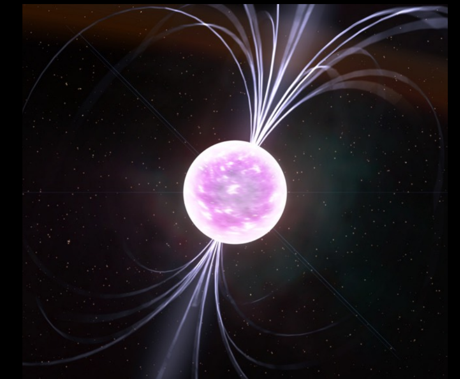
Pulsars
