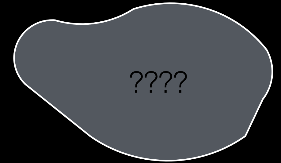
Pulsars
