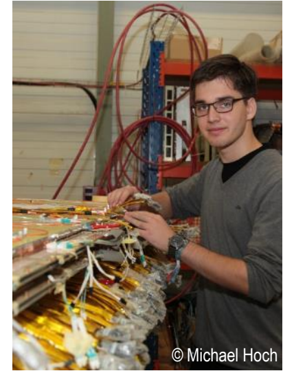
Forschungsprojekte (Standorte/CERN)
