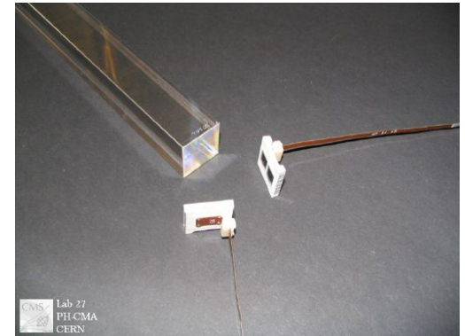
Кристал от оловен волфрамат и лавинни фотодиоди, използвани в ECAL на CMS
