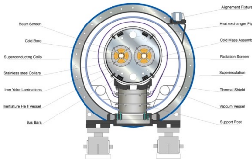
LHC gyorsító
