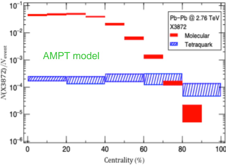
PRL 136, 012301 (2021)
