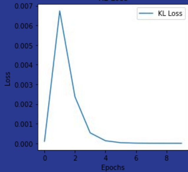
KL Loss
