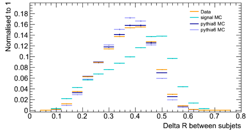
com fox wolfram 1
