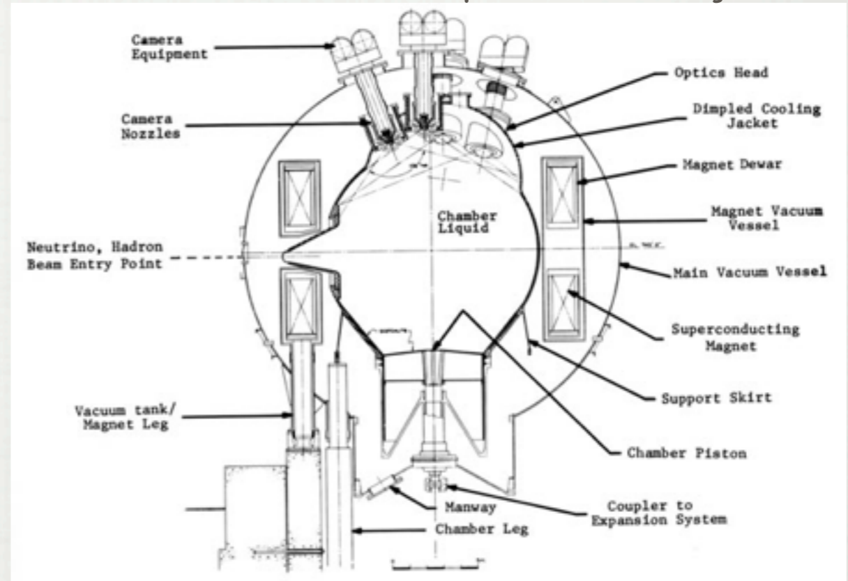
Fermilab 15' (4.6m) köpük odasının çizimi
