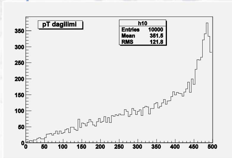
❖ Muon pT dağılımı(spektrumlu)
