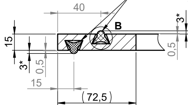
COUPE A-A ECHELLE 1 : 2
