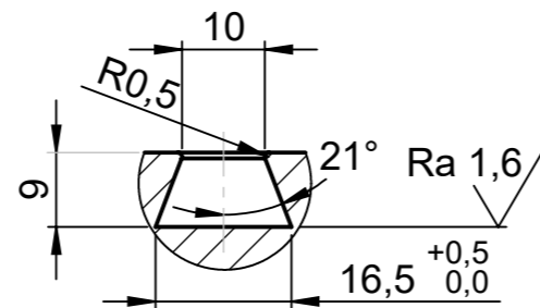
DÉTAIL B ECHELLE 1 : 1
