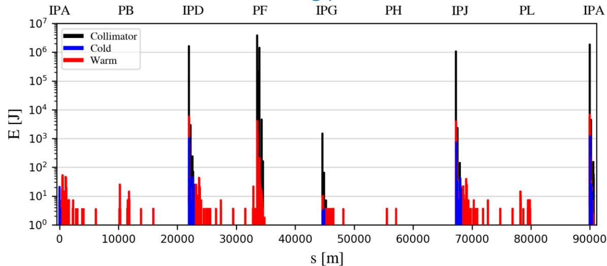
0deg phase
