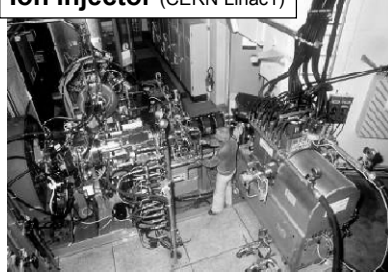
Ion injector (CERN Linac1)
