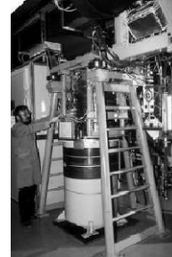
3 GHz klystron (CERN LPI)
