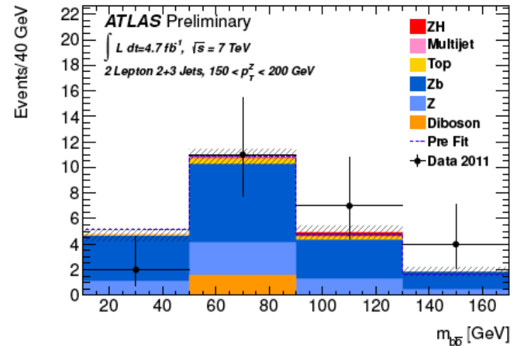
(d) 150 < p_T^Z < 200 \text{ GeV}
