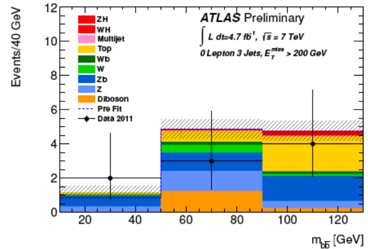
(f) E_T^{\text{miss}} > 200 \text{ GeV} , 3 jets
