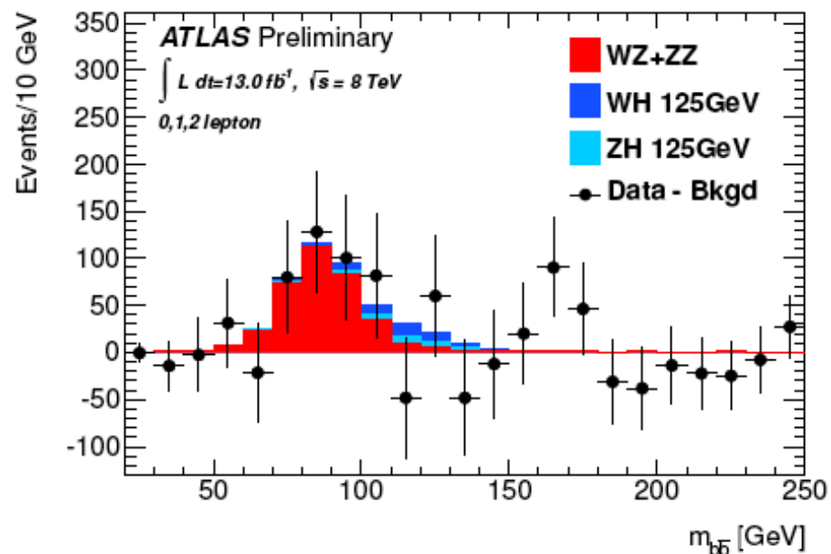
(b) \sqrt{s} = 8 \text{ TeV}
