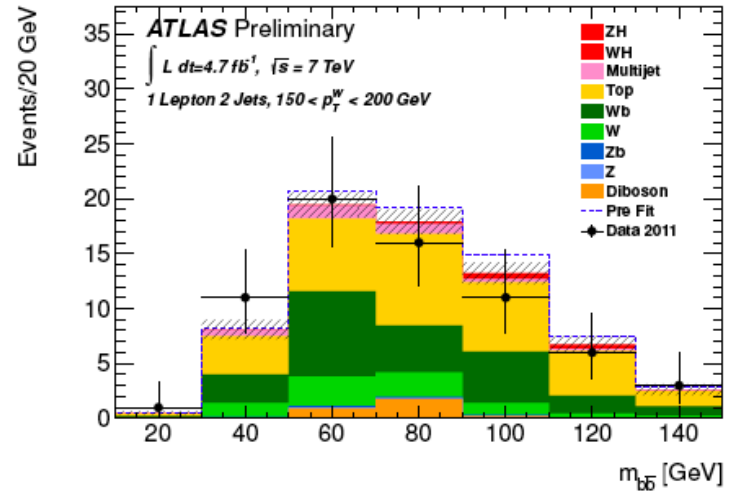
(d) 150 < p_T^W < 200 \text{ GeV}
