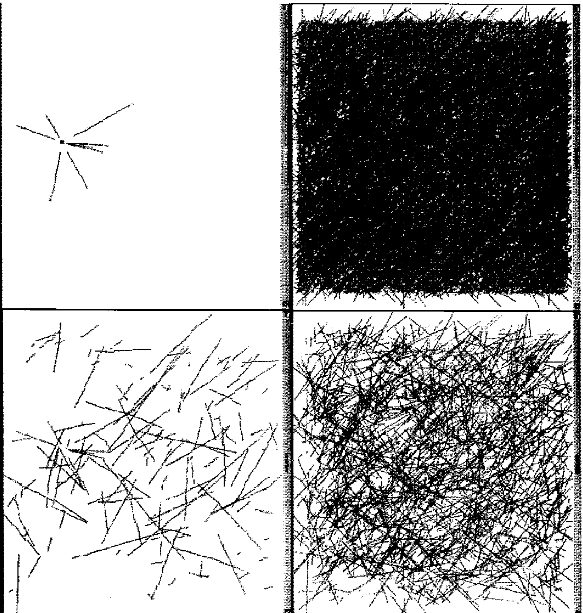
図 5.12: net scan 反応点探索の各段階(左上から時計回り)。1) 読み込んだ全ての飛跡 ( 5 \times 5 \text{mm}^2 )、2) 測定領域を突き抜けている飛跡の排除、3) 低運動量の飛跡の排除、4) 一点 ( 4\mu\text{m} 以内) 収束している飛跡
