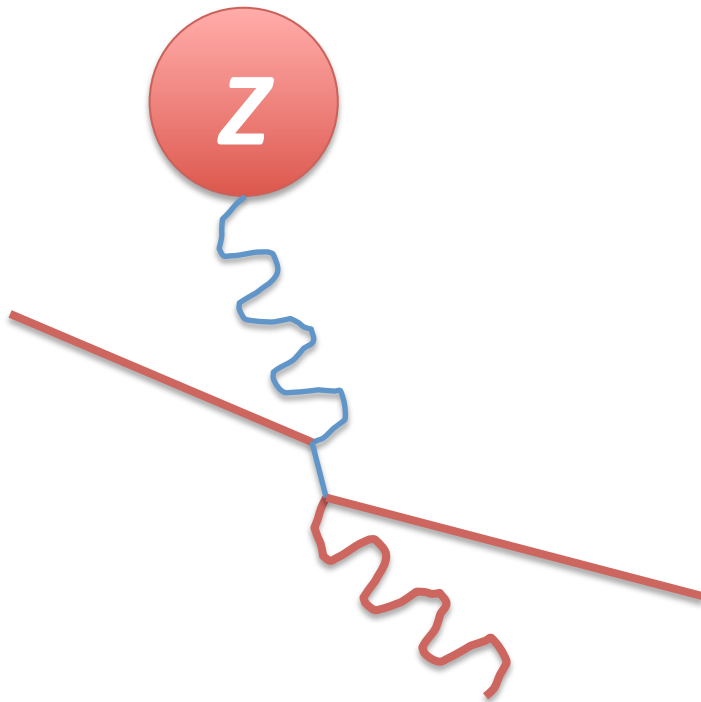
Bremsstrahlung
