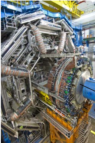
Un calorimètre d'extrémité et l'aimant toroidal central
