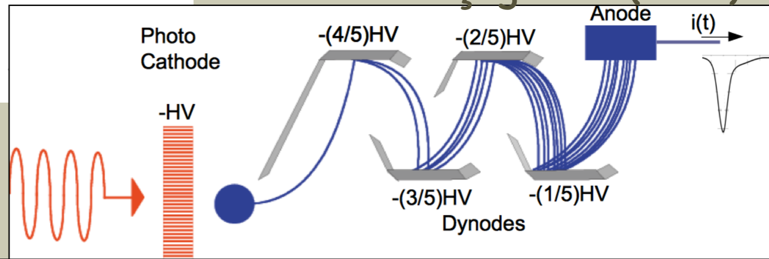
fotoçoğaltıcı (PMT)
