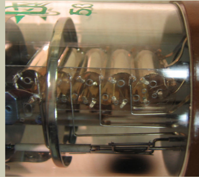
fotoçoğaltıcı (PMT)
