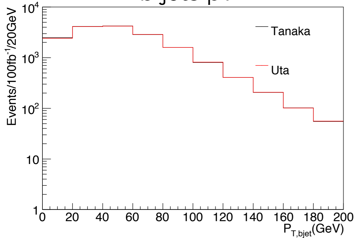
b-jets pT
