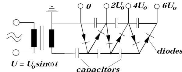
Κύκλωμα Greinacker
