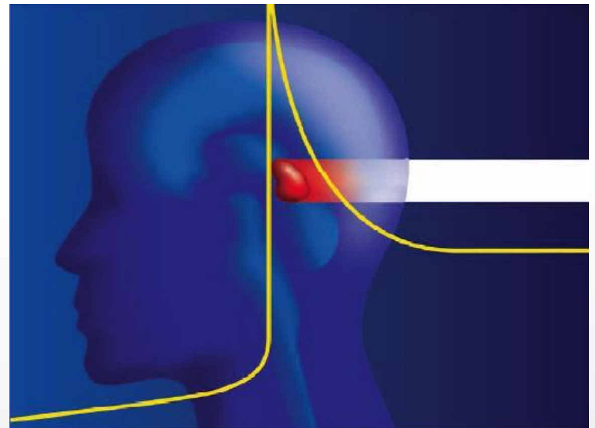
Antiprotons
