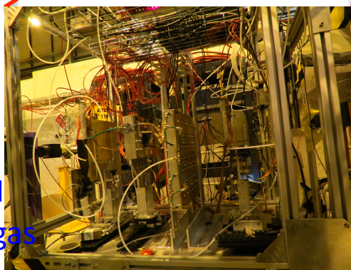
DHCAL-THGEM
