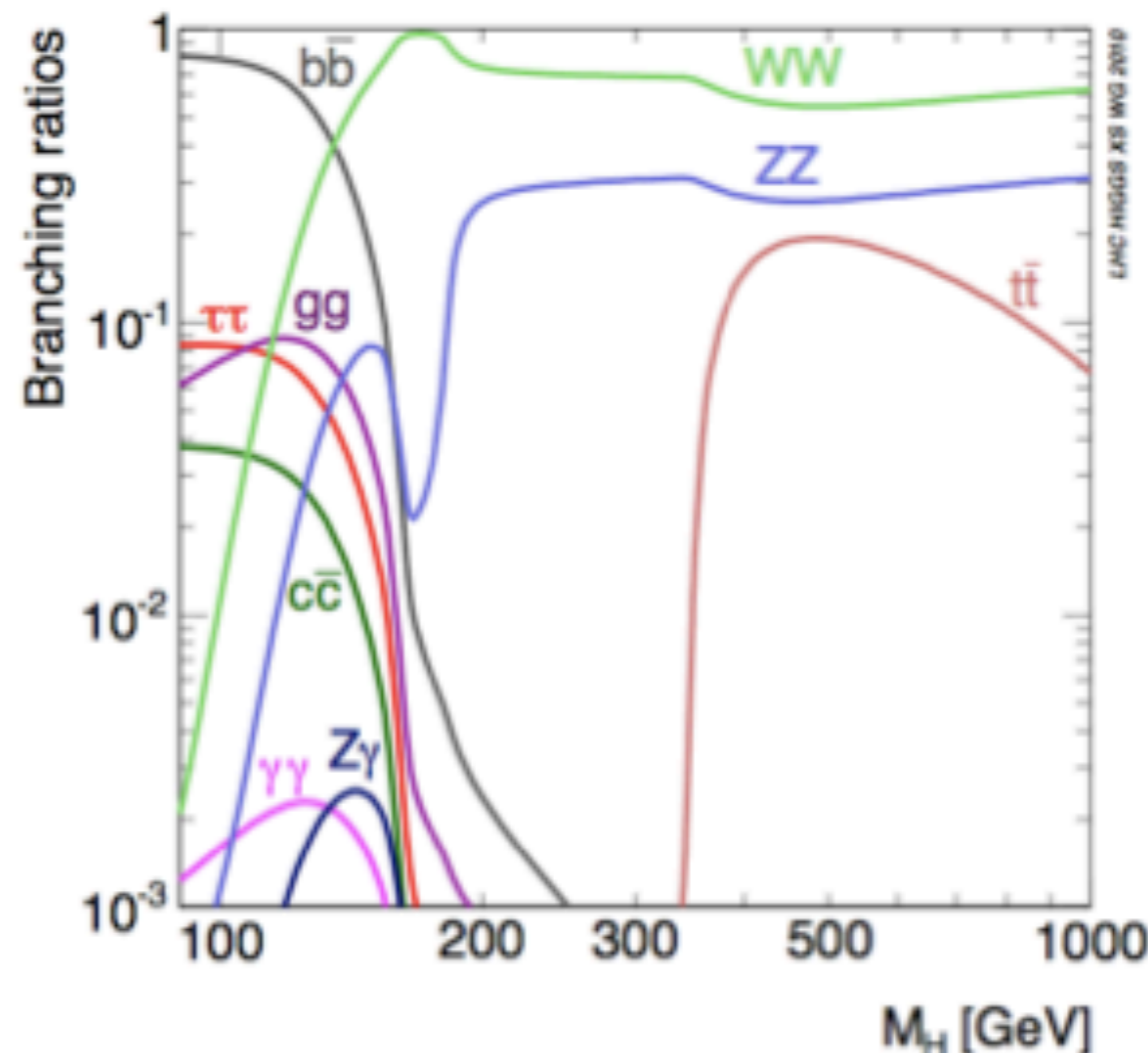
VH
