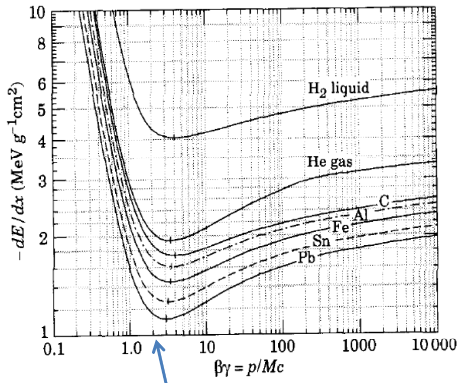
Minimal ionisierendes Teilchen MIP
