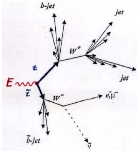
NACHWEIS ANHAND DER ZERFALLSPRODUKTE
