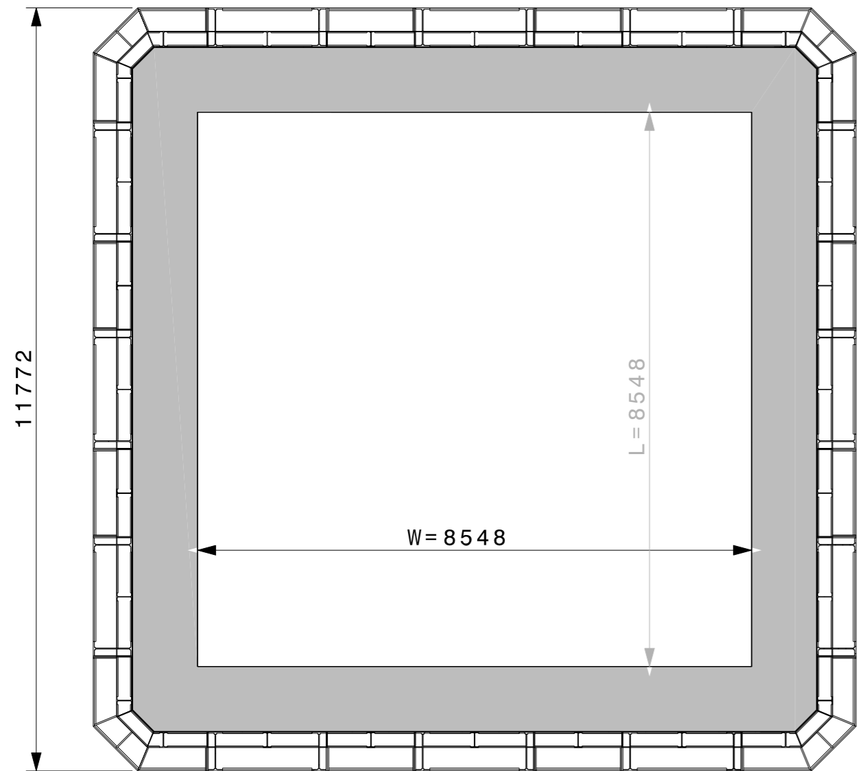
C-C 1:80
