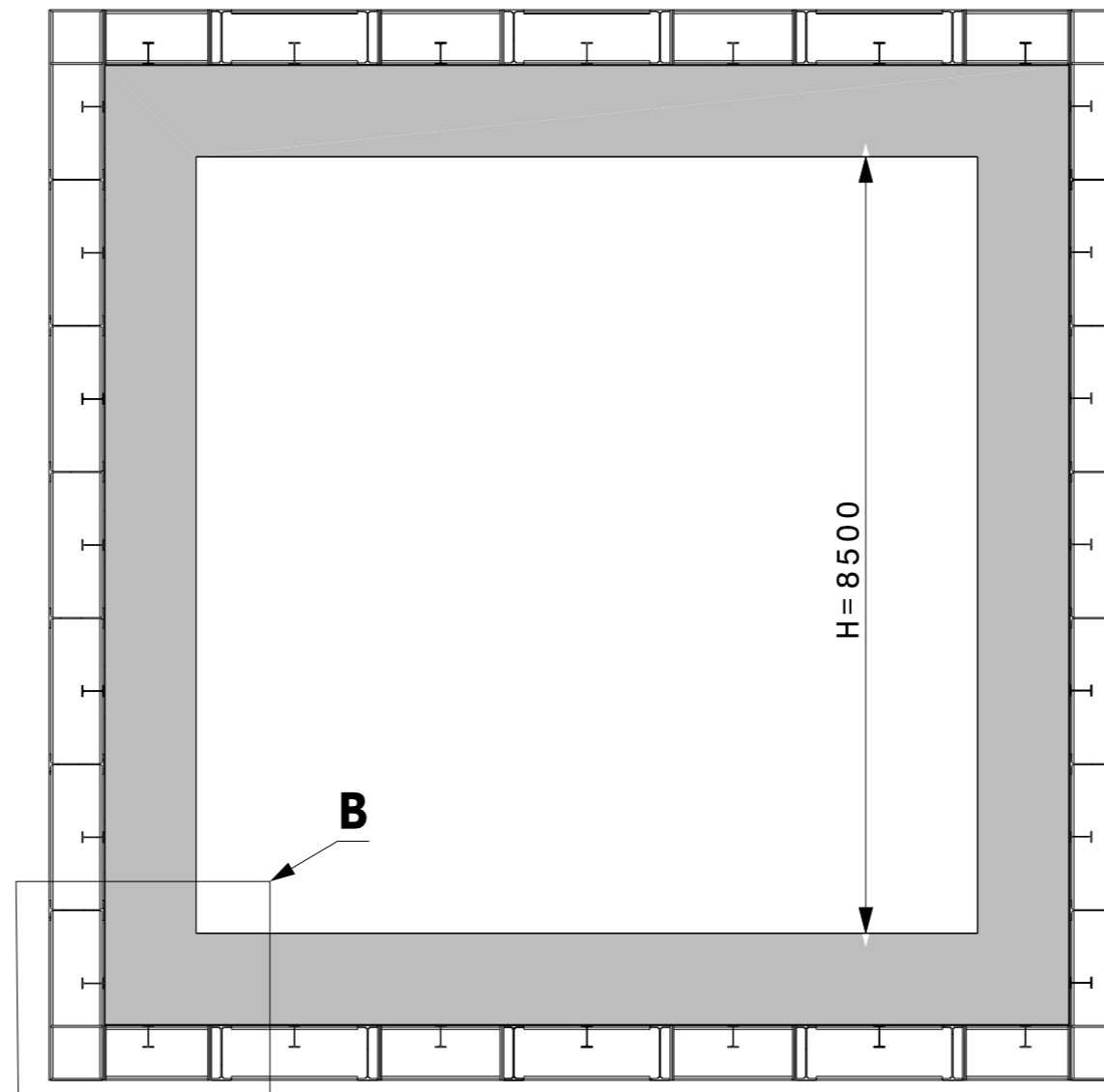
A-A 1:80
