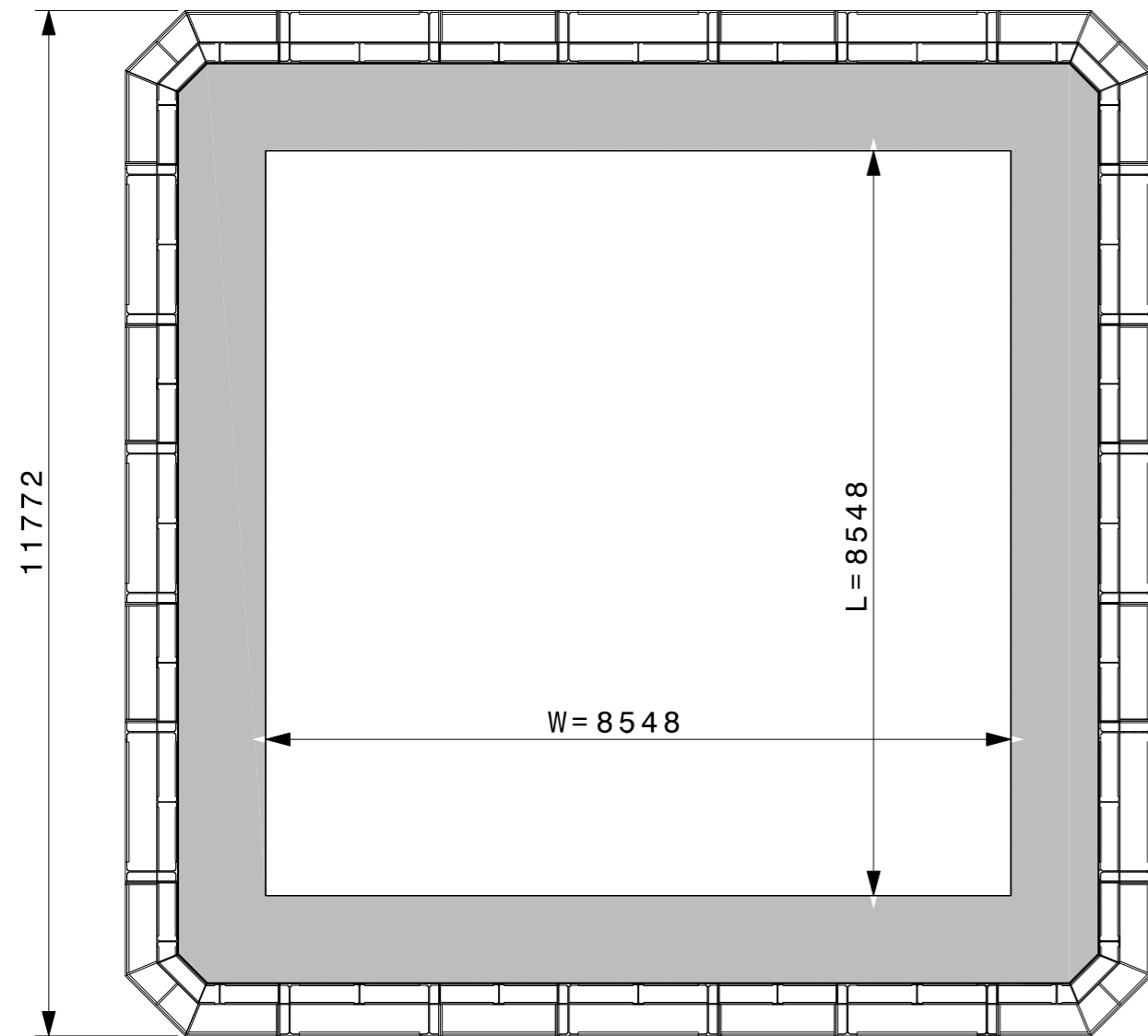
C-C 1:80
