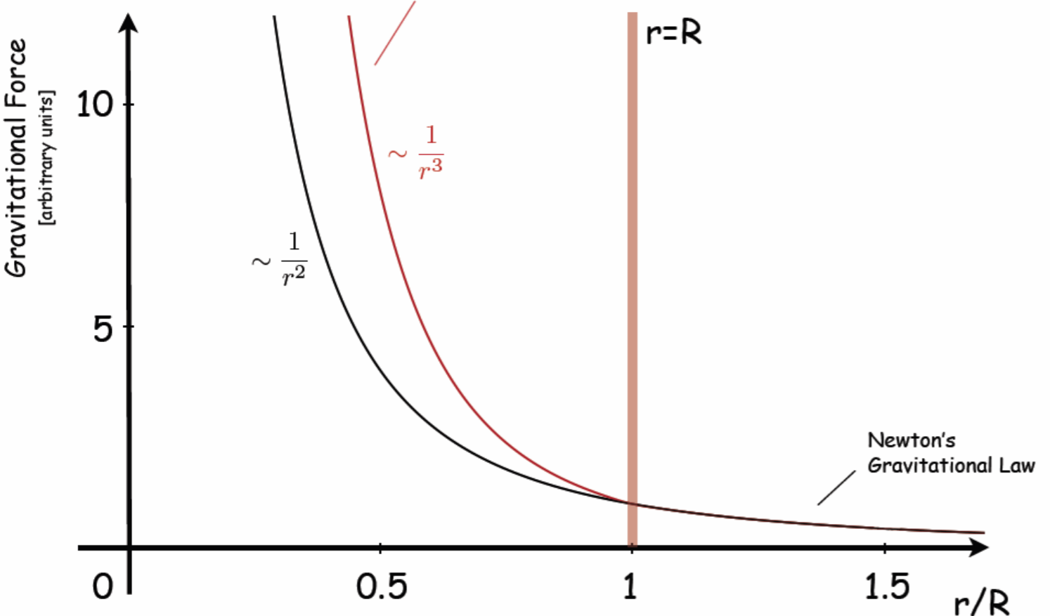
Gravitation in 4 Raumdimensionen
