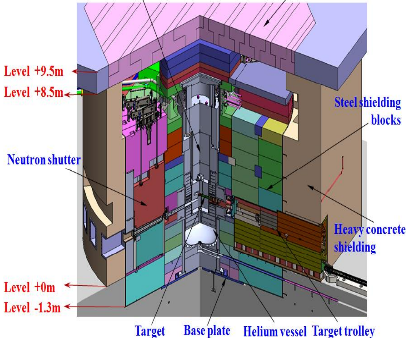
Moderator&Reflector plug
