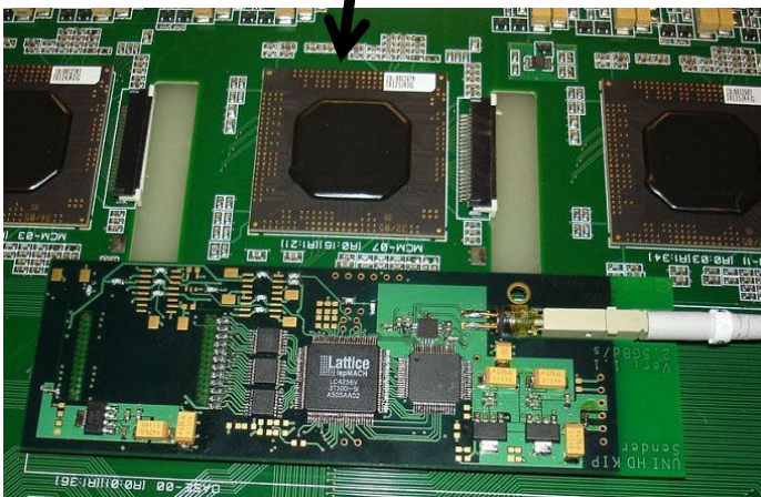
Eine mit Elektronik bestückte Auslesebox
