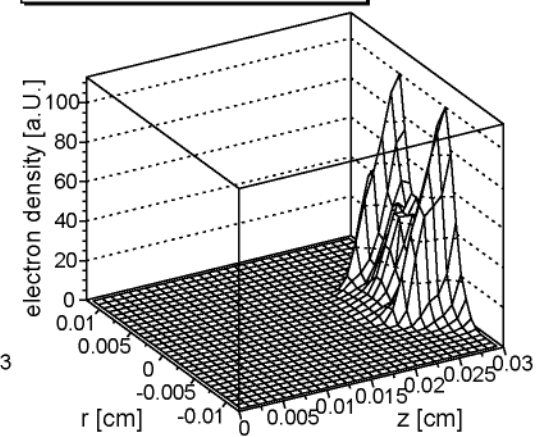
f) t=1.52\text{ns} ; 50399 electrons
