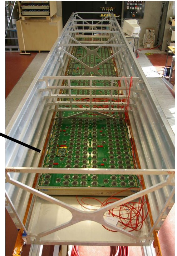
Ein TRD Supermodul in Bau Die erste der 6 Detektorebenen wird installiert.
