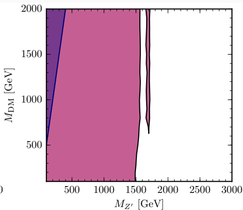
(d) g_q = 0.375 and g_{DM} = 0.25
