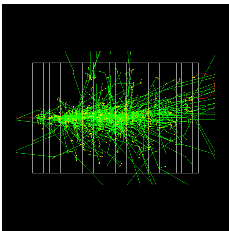
1 GeV енергия в ЕМ калориметър
