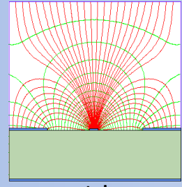
Микрострип
