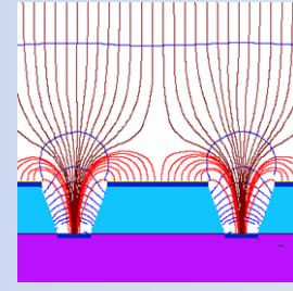
GEM газовый электронный усилитель
