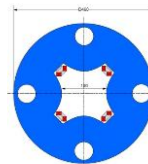
Skew quadrupole (INFN)
