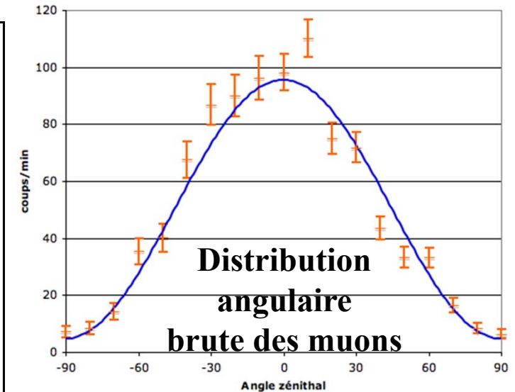
Figure 4 : Distribution zénithale des muons
