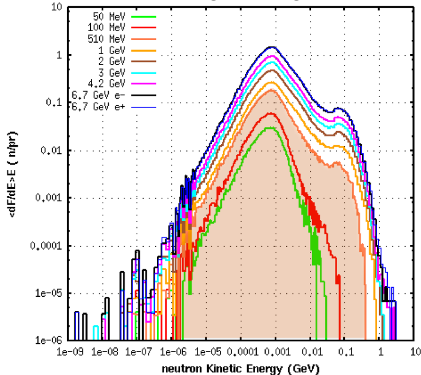
Tungsten target
