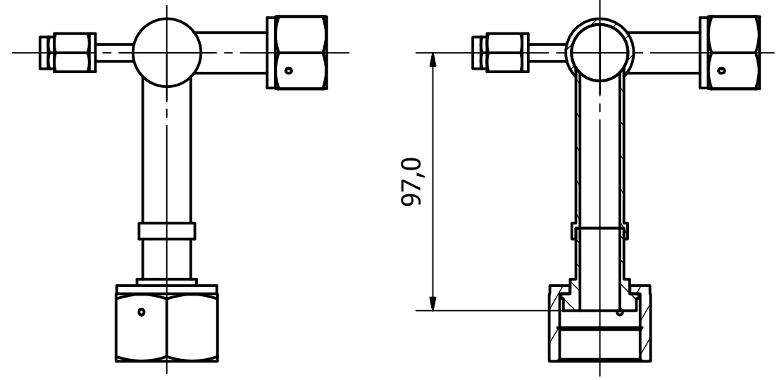
C-C ( 1 : 2 )
