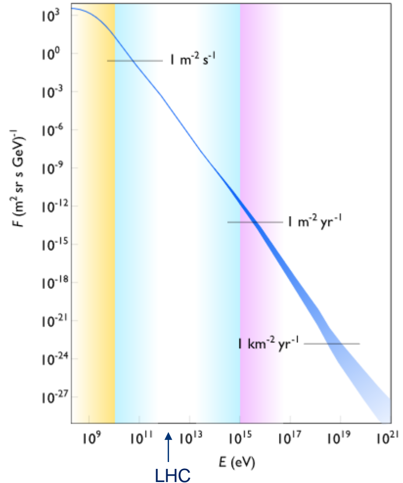
Energieverteilung von Kosmischer Strahlung
