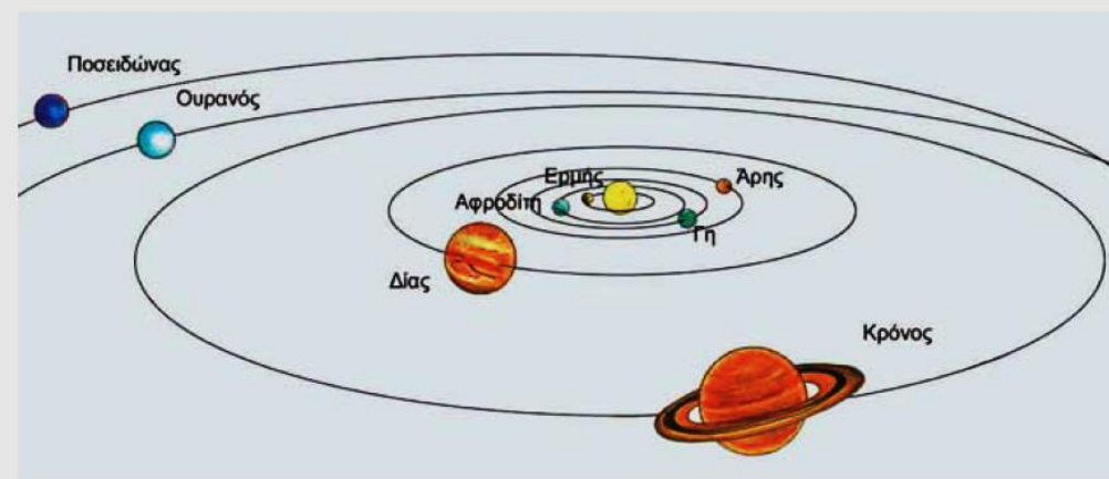
Εικόνα 6.1: Οι πλανήτες
